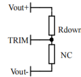
电压下调: 在Trim和输出正之间增加电阻Rdown
