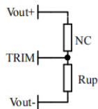
电压上调: 在Trim和输出负之间增加电阻Rup
